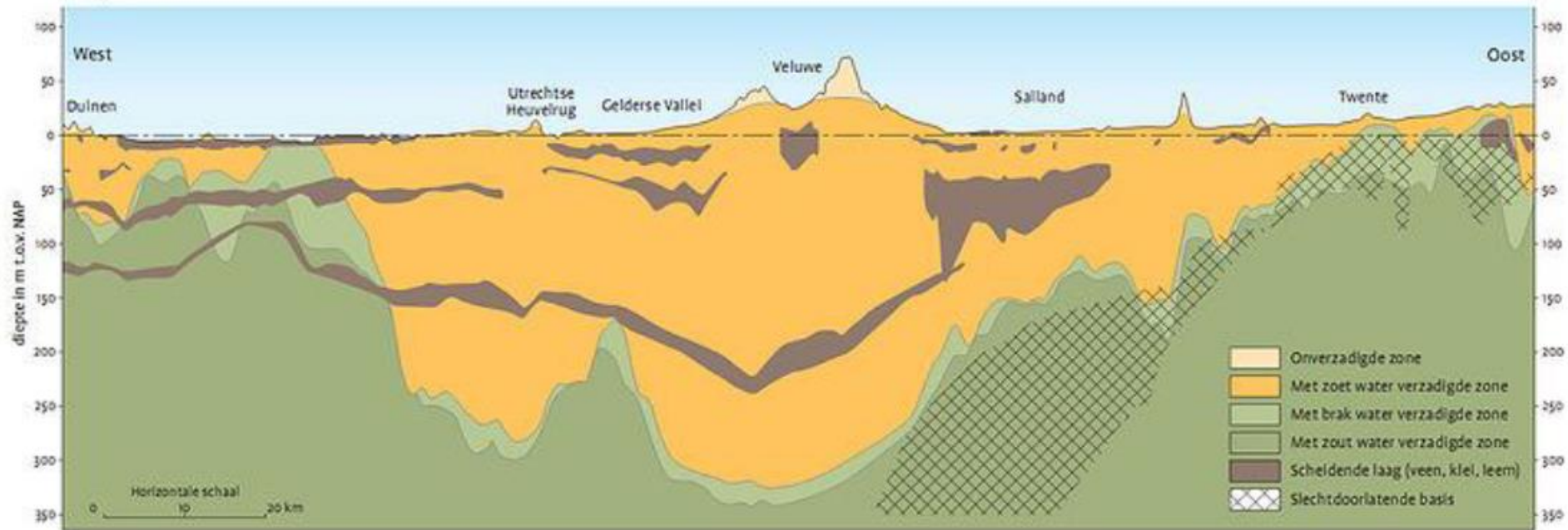
Dwarsprofiel
